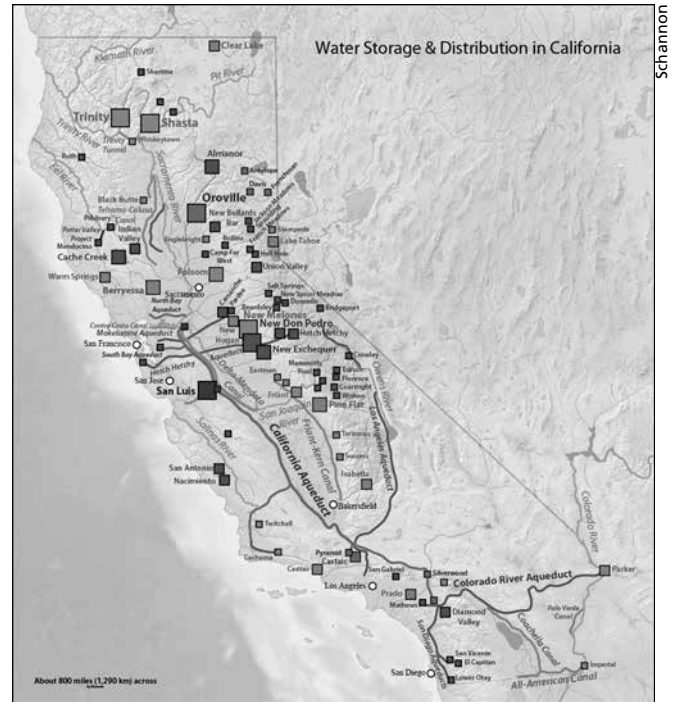
Le système de stockage et de distribution de l'eau en Californie. Les carrés représentent les différentes infrastructures, qui peuvent être de gestion publique ou privée. On y trouve aussi les aqueducs et rivières évoqués dans l'article.
