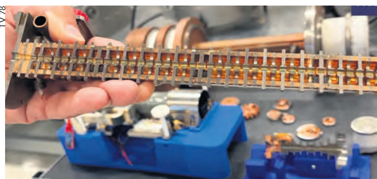
Tube électronique produit dans l'usine Thales à Vélizy.
